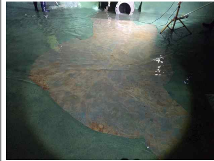
<배수지 2지 바닥슬래브 도장박락>
