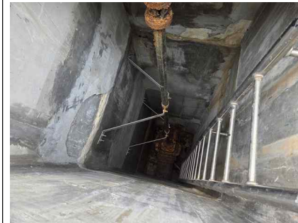
<제수밸브실 배관부식>
